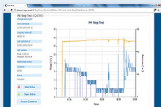
Gráficos comprimidos de caudal en cada cierre de válvula.
